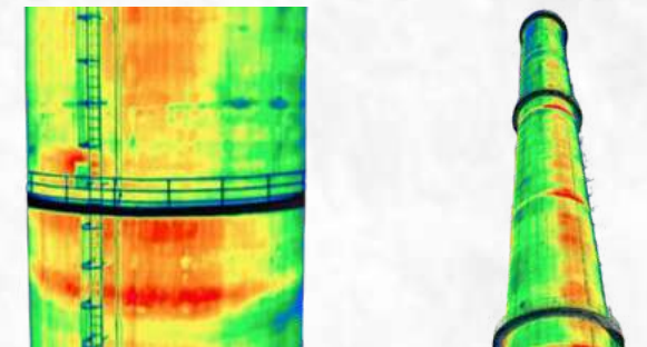
Termografía (Chimenea)
